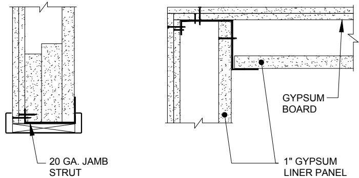
6 JAMB DETAIL SECTION C-C
