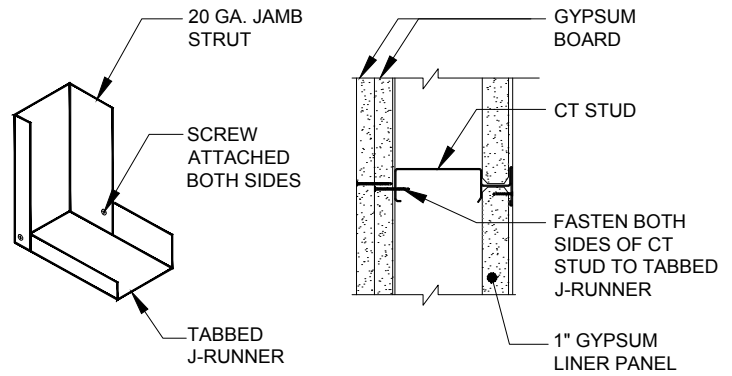
3 JAMB DETAIL
