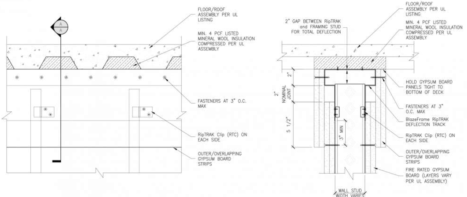
SECTION A-A
