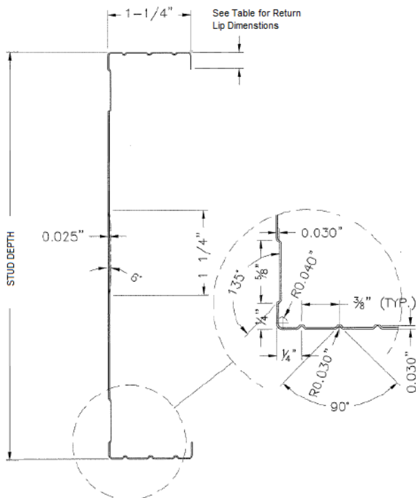
3-1/2\", 3-5/8\", 4\", 5-1/2\" & 6\" Studs
